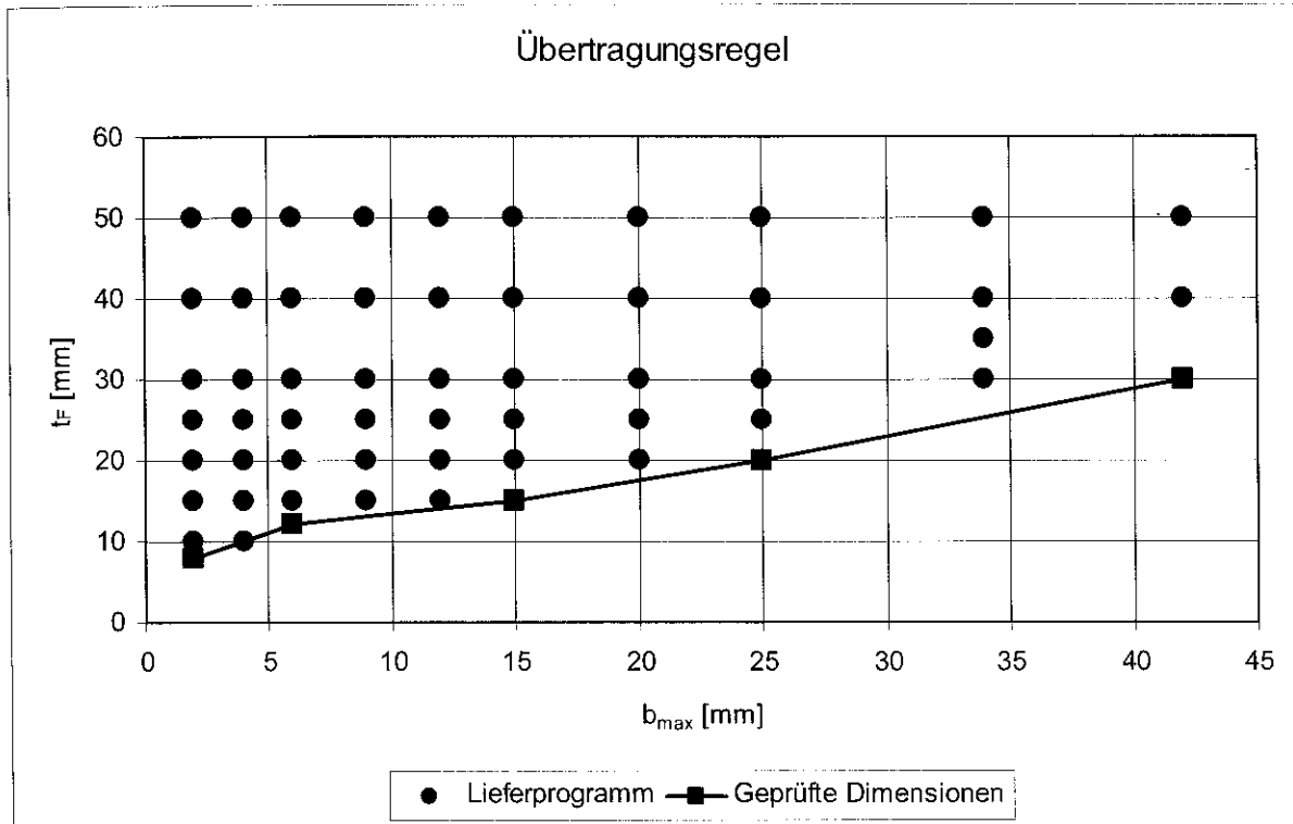
Bild 2 Anwendung der Übertragungsregel nach DIN 18542, Abschnitt 7, Bild 4
